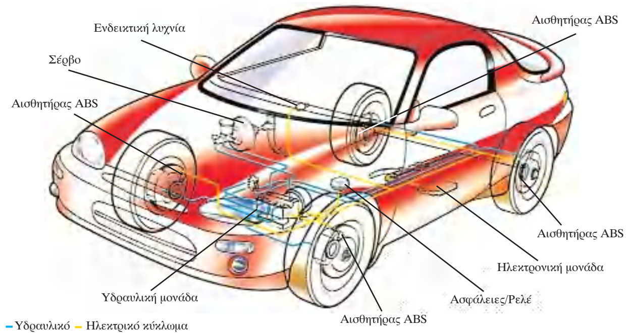
Σχ. 21.1 Ηλεκτρικό και υδραυλικό κύκλωμα ABS.
