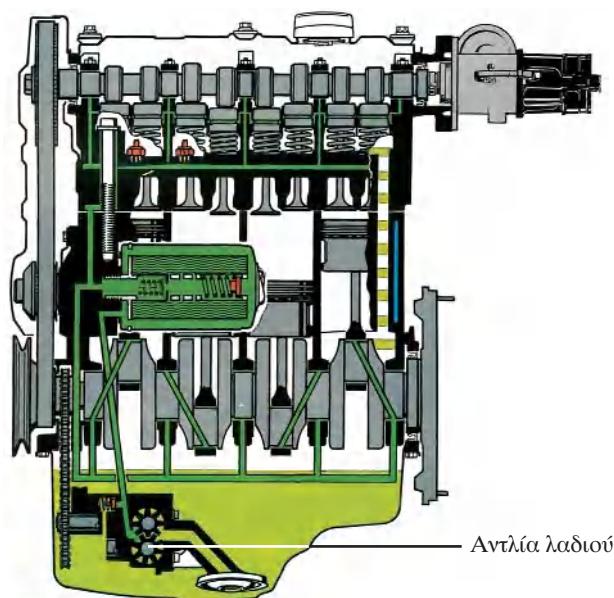
Σχ. 3 Σύστημα λιπάνσεως.
