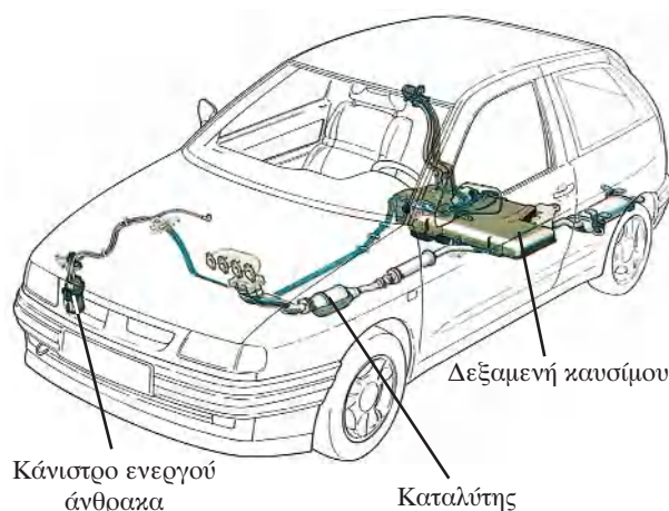
Σχ. 7 Διάταξη αντιρρυπαντικών συστημάτων.
